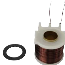
138940 Solenoid Coil 24 V, ID 21.10, OD 46.75
